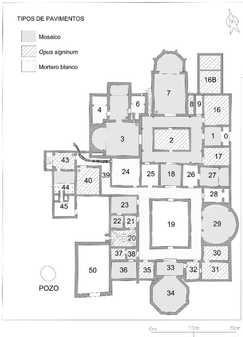
Figura 3. Planta de la pars urbana en su inicio. (Dibujo: E. Martínez).
